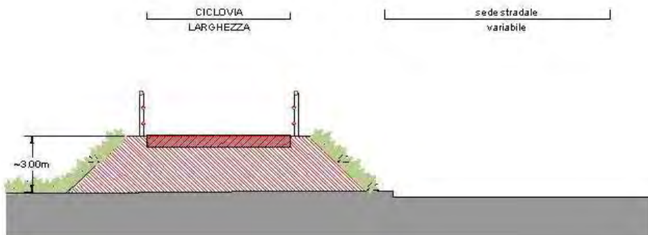
H5 - REALIZZAZIONE CICLOVIA IN RILEVATO
