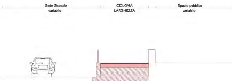
M6 - RAMPA COLLEGAMENTO SPAZIO PUBBLICO A QUOTA VARIABILE
