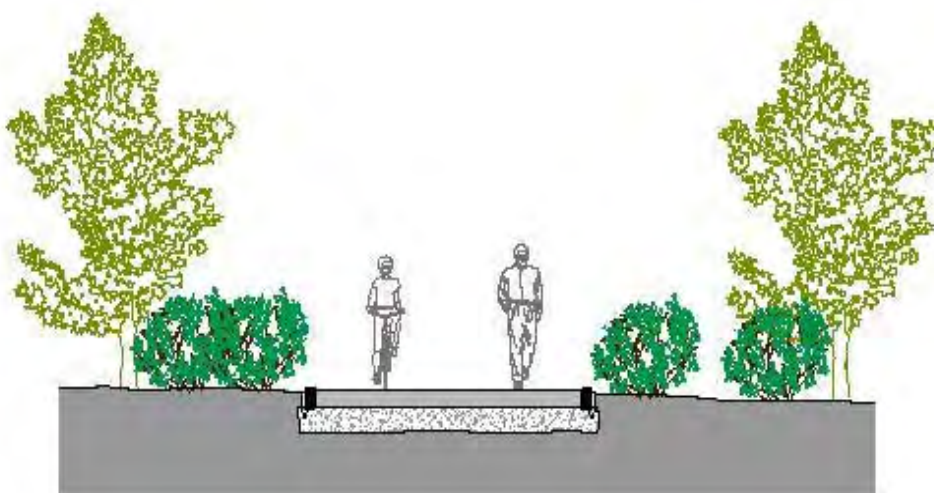
L3 - PISTA CICLABILE SU TRATTI SABBIOSI CON SOTTOFONDO DRENANTE E PAVIMENTAZIONE IN STABILIZZATO A CALCE
