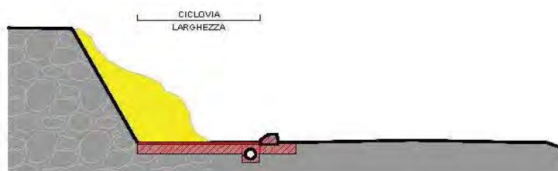
17 - REALIZZAZIONE CICLOVIA IN SEDE PROPRIA CON SCAVO A MONTE IN ROCCIA
