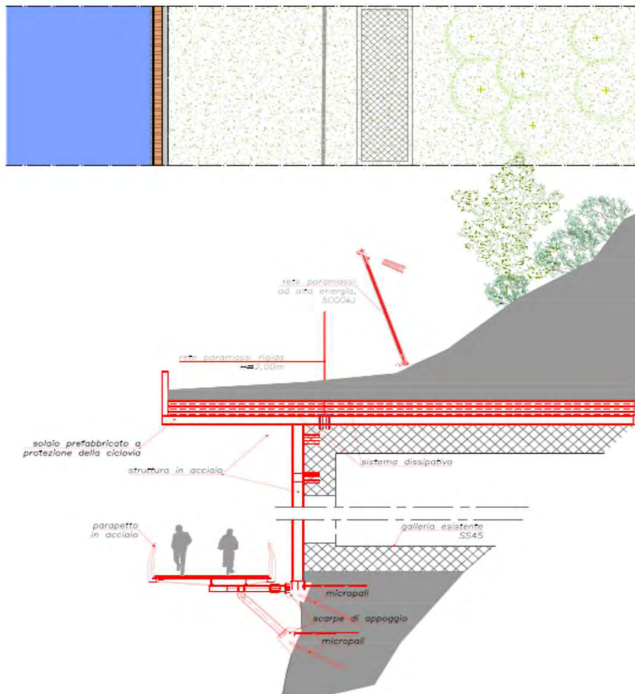
N13 - CICLOVIA SU MENSOLA A SBALZO AFFIANCATA A SS/SR IN GALLERIA ARTIFICIALE
