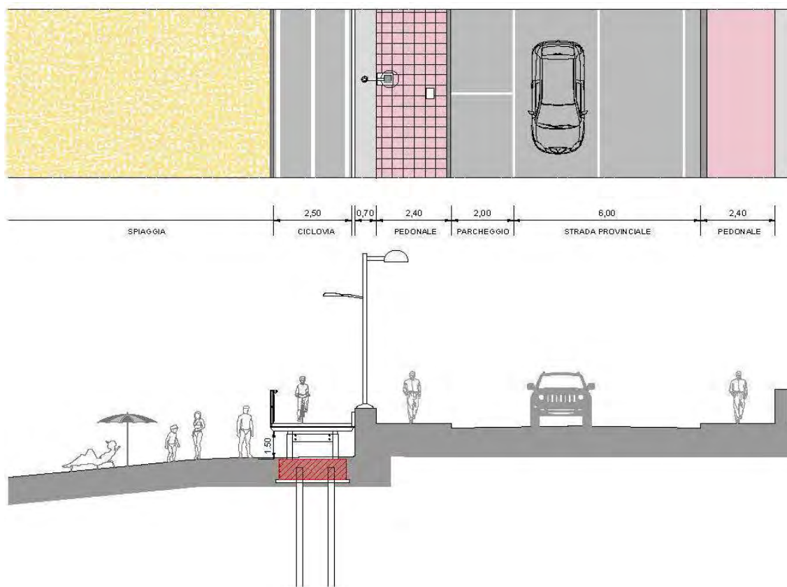
N2 - CICLOVIA LUNGOMARE su portali L= 2,50m
