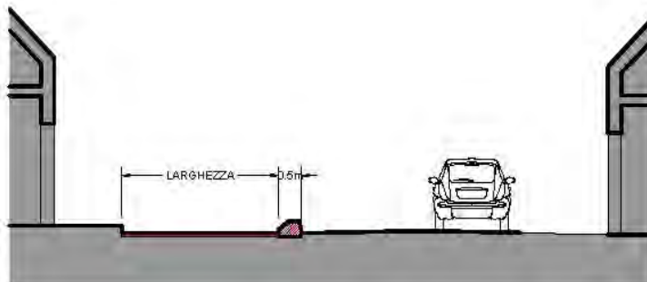
G9 - REALIZZAZIONE CICLOVIA RICAVATA SU PIATTAFORMA STRADALE CON CORDOLO DI SEPARAZIONE (2)
