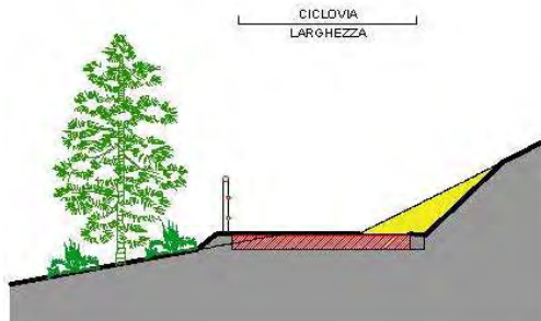
15 - PISTA CICLOPEDONALE CON ALLARGAMENTO SENTIERO ESISTENTE
