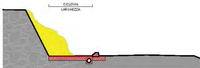
I7 - REALIZZAZIONE CICLOVIA IN SEDE PROPRIA CON SCAVO A MONTE IN ROCCIA
