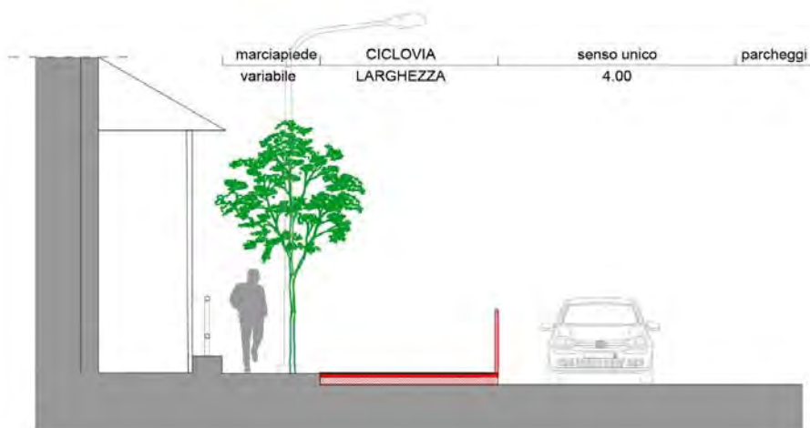
O15 -NUOVA PISTA CICLABILE IN ALLARGAMENTO A MARCIAPIEDE ESISTENTE
