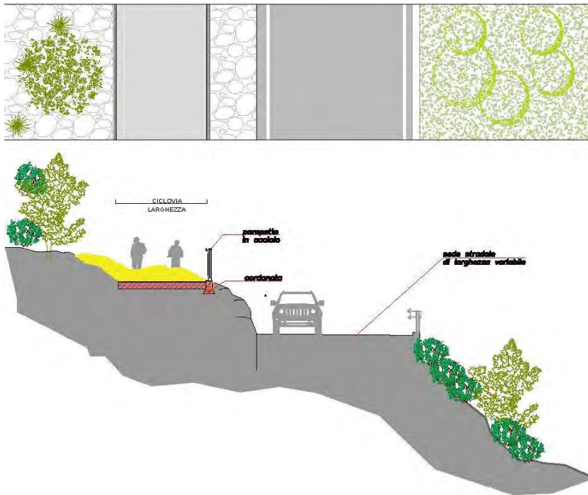
M5 - CICLOVIA SU RILEVATO ROCCIOSO
