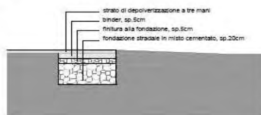
Dettaglio scala 1:25
