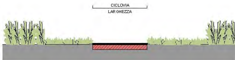
G1 - NUOVA CICLOVIA A PIANO CAMPAGNA
