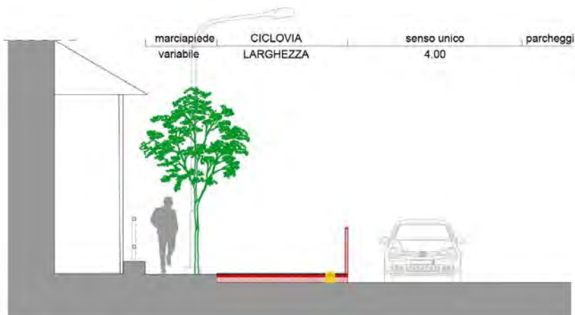
O32 -ADEGUAMENTO PISTA CICLABILE ESISTENTE E GRIGLIA ALBERI ESISTENTI
