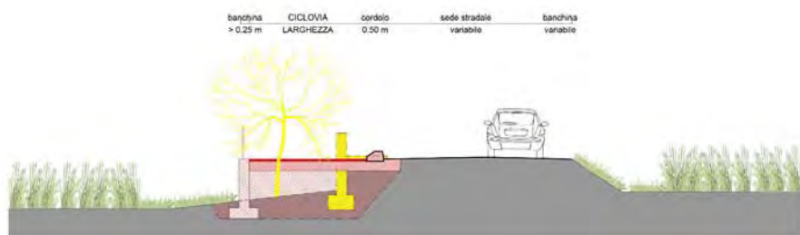
M7 - ALLARGAMENTO PISTA CICLABILE ESISTENTE IN SEDE PROPRIA CON ARRETRAMENTO MURO DI SOSTEGNO
