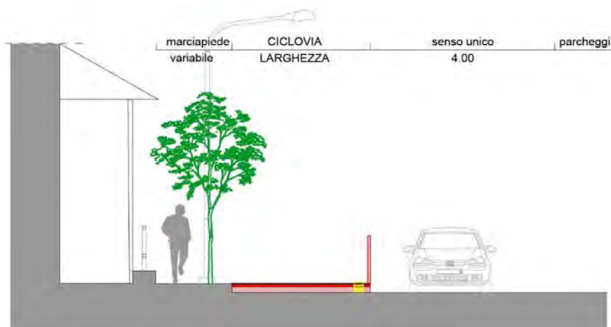
O30 -ADEGUAMENTO PISTA CICLABILE ESISTENTE (tipo 1)
