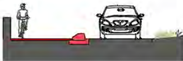
O18 - PERCORSO CICLOVIA CON CORDOLO SEPARATORE
