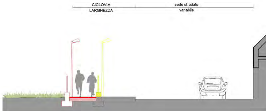
L11 - ALLARGAMENTO PISTA CICLABILE CON PAVIMENTAZIONE IN BETONELLE E SPOSTAMENTO OPERE INTERFERENTI
