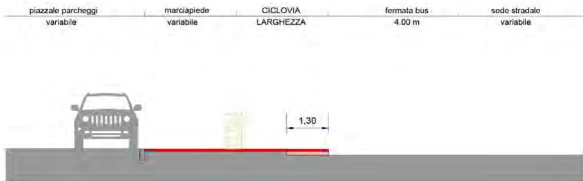
O14 - ADEGUAMENTO CICLOVIA A QUOTA MARCIAPIEDE
