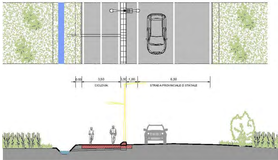
G3 - REALIZZAZIONE CICLOVIA IN AFFIANCAMENTO CON CORDOLO E FOSSO
