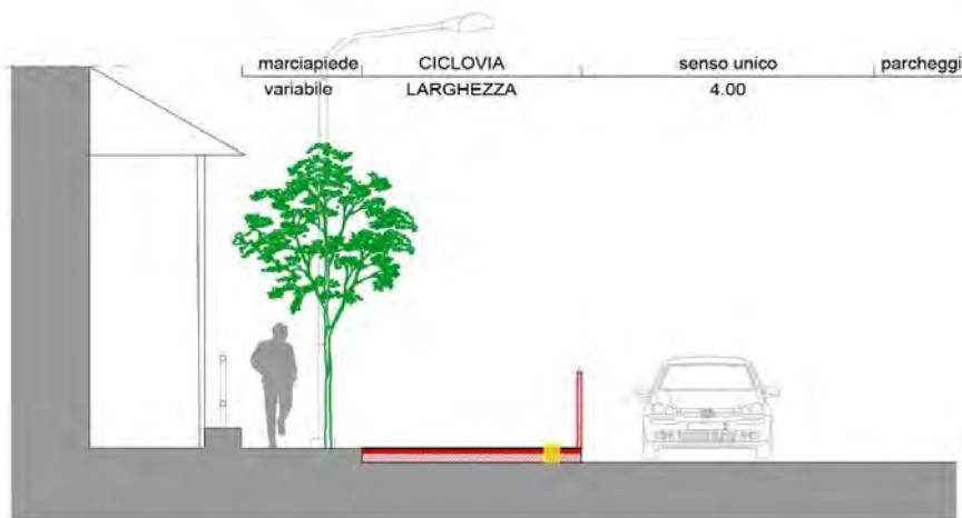
O31 - ADEGUAMENTO PISTA CICLABILE ESISTENTE (tipo 2)
