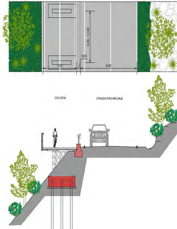
N3 - CICLOVIA LATO STRADA CON BARRIERA STRADALE su setti L=3,50
