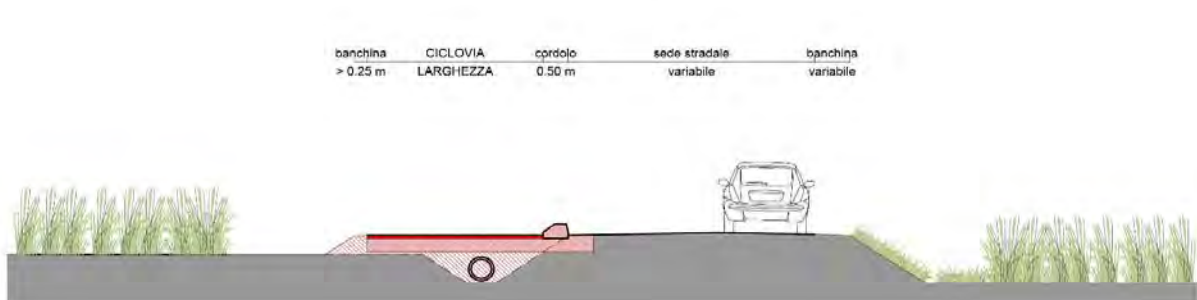
G16 - NUOVA CICLOVIA IN AFFIANCAMENTO CON CORDOLO E TOMBINATURA FOSSO
