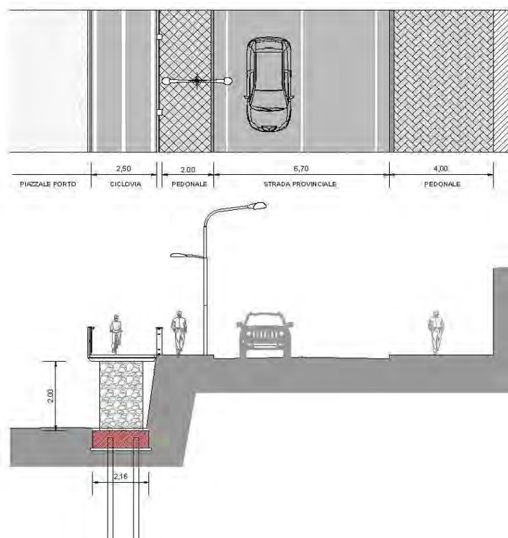
N1 - CICLOVIA LUNGOMARE su setti L= 2,50m
