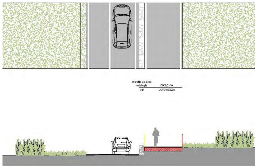
G10 - REALIZZAZIONE CICLOVIA CON RISANAMENTO MURI A SECCO
