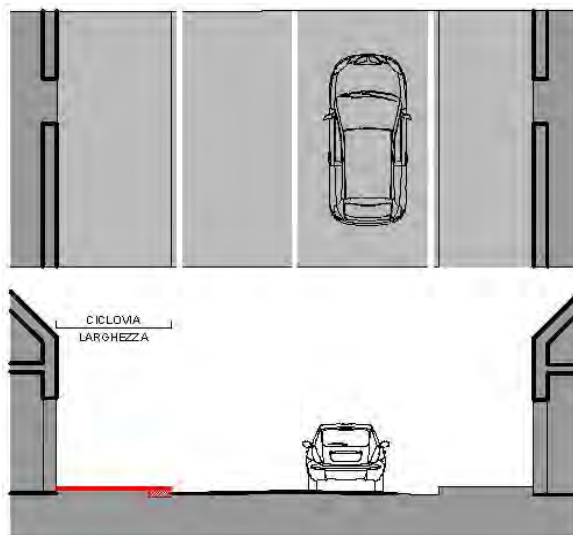
E3 - ALLARGAMENTO PERCORSO CICLABILE RIALZATO (2,50-3,50)
