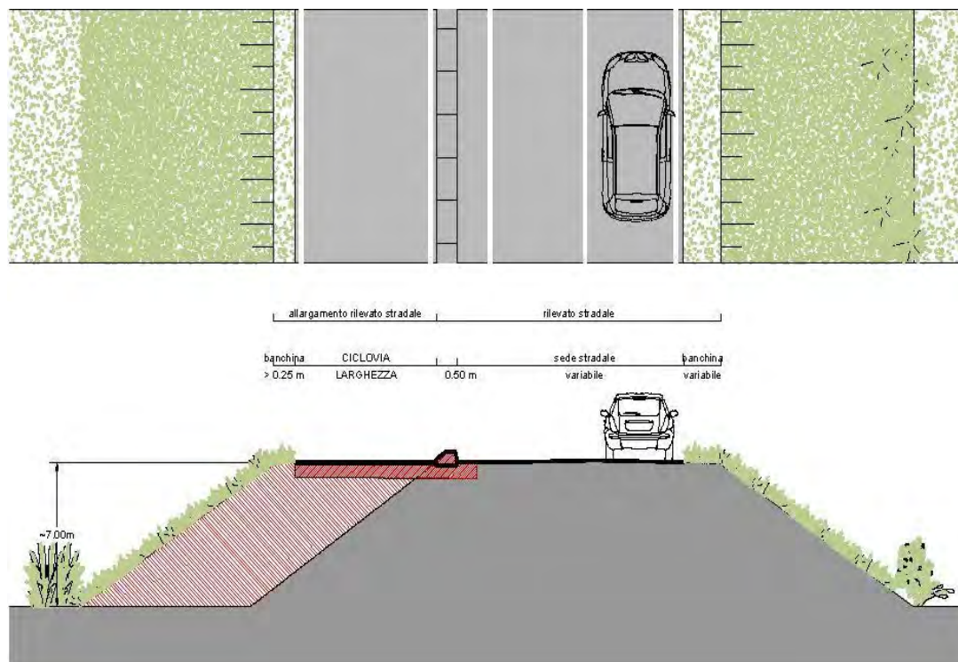
H3 REALIZZAZIONE CICLOPEDONALE IN SEDE PROPRIA CON CORDOLO (Strada Alto Traffico) H < 7,00
