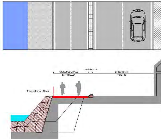
M3 - CICLOVIA LUNGOMARE IN SEDE PROPRIA CON SCOGLIERA
