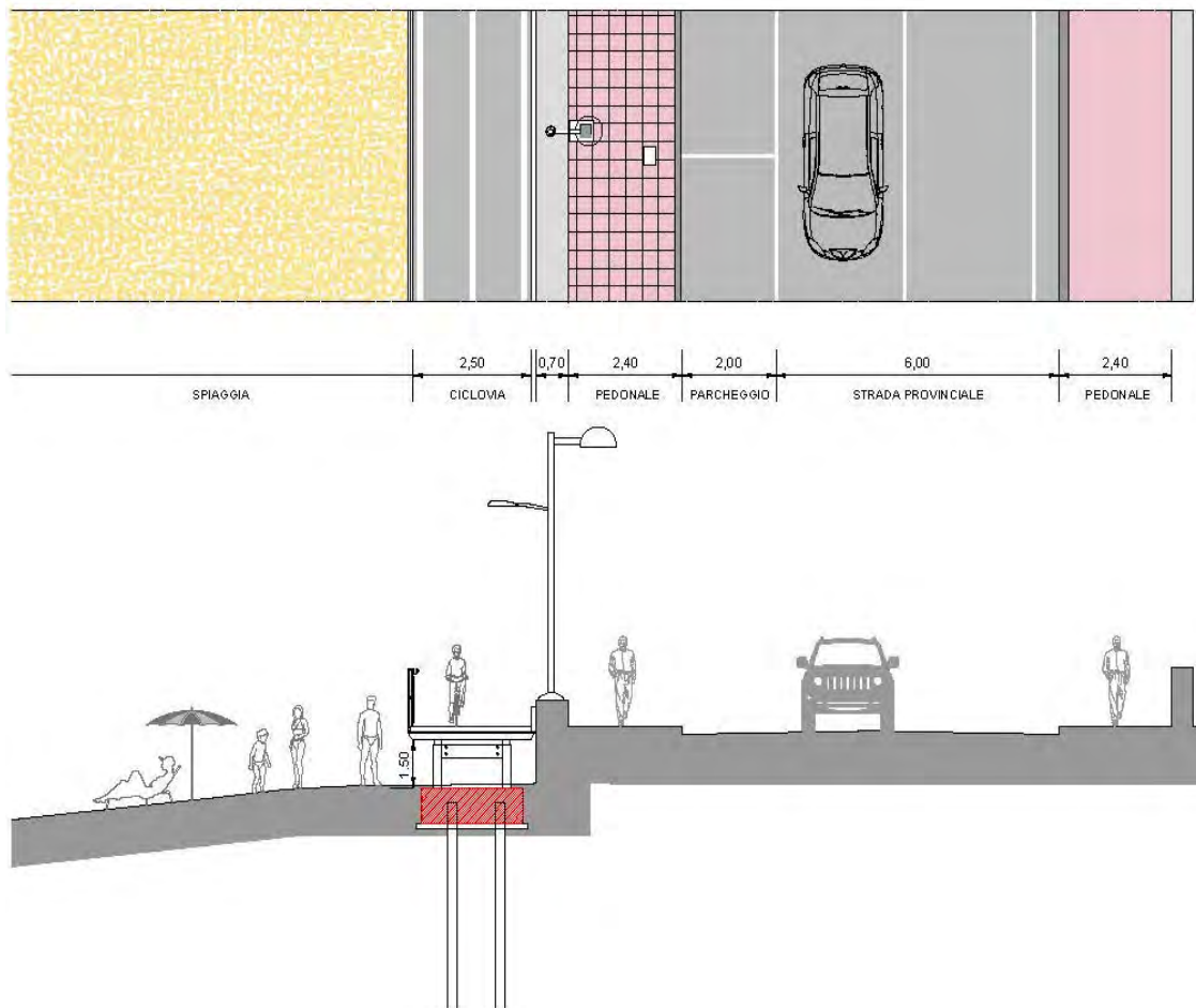
N2 - CICLOVIA LUNGOMARE su portali L= 2,50m
