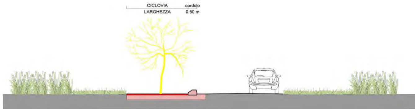
G17 - NUOVA CICLOVIA IN AFFIANCAMENTO CON CORDOLO E TAGLIO PIANTE
