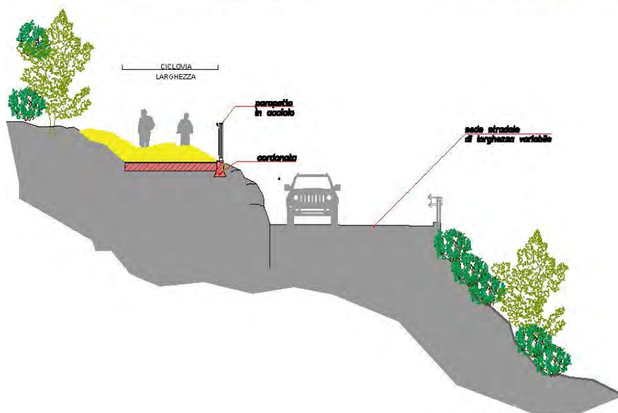
M5 - CICLOVIA SU RILEVATO ROCCIOSO
