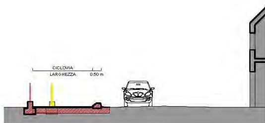
M1 - ALLARGAMENTO PISTA CICLABILE ESISTENTE IN SEDE PROPRIA CON ARRETRAMENTO RECINZIONI
