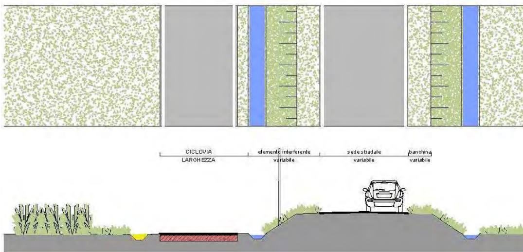
G2 - NUOVA CICLOVIA A PIANO CAMPAGNA CON SPOSTAMENTO FOSSO
