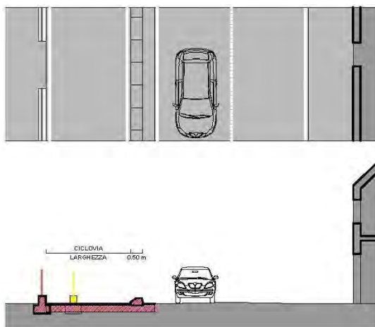
G4 - NUOVA CICLOVIA AMBITO URBANO CON SPOSTAMENTO RECINZIONE
