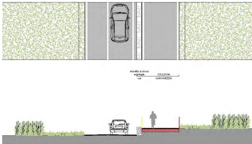
G10 - REALIZZAZIONE CICLOVIA CON RISANAMENTO MURI A SECCO
