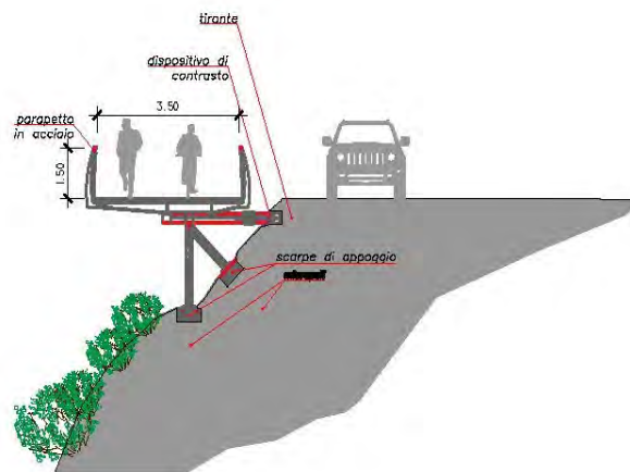
N12 - CICLOVIA SU MENSOLA A SBALZO SU FRONTE ROCCIOSO
