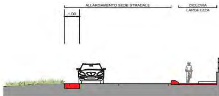
O17 - PERCORSO CICLOVIA IN SEDE PROPRIA CON SPOSTAMENTO SEDE STRADALE
