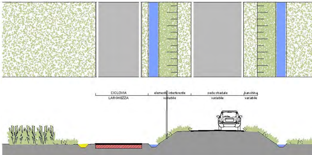
G2 - NUOVA CICLOVIA A PIANO CAMPAGNA CON SPOSTAMENTO FOSSO
