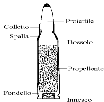
Sezione di una cartuccia per fucili a canna rigata
