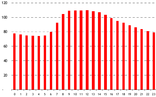
Profilo "centro commerciale" allacciato in MT (800 MWh/anno) Profilo di consumo medio giornaliero (kWh)
