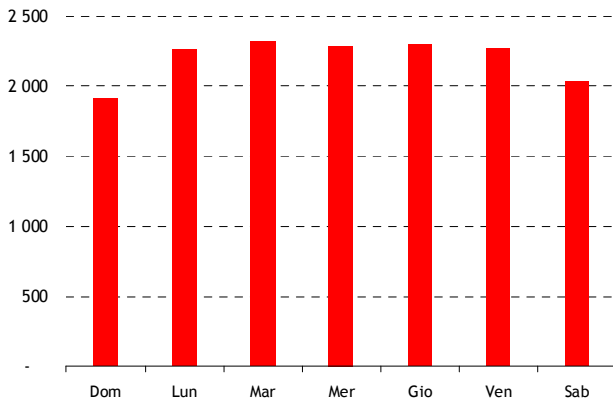
Profilo "centro commerciale" allacciato in MT (800 MWh/anno) Profilo di consumo medio settimanale (kWh)
