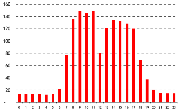
Profilo "impresa manifatturiera" allacciata in MT (600 MWh/anno) Profilo di consumo medio giornaliero (kWh)
