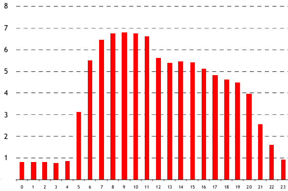
Profilo "commercio" allacciato in BT (35 MWh/anno) Profilo di consumo medio giornaliero (kWh)
