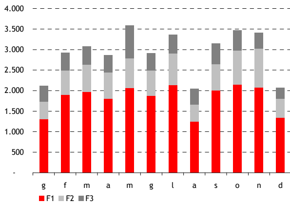
Profilo "commercio" allacciato in BT (35 MWh/anno) Profilo di consumo medio mensile (kWh)
