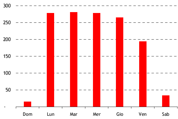
Profilo "artigiano" allacciato in BT (70MWh/anno) Profilo di consumo medio settimanale (kWh)
