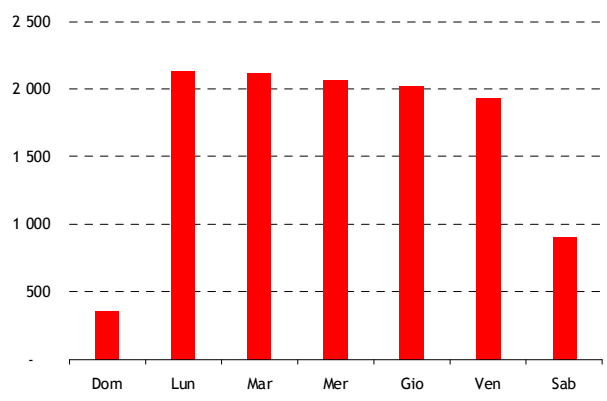
Profilo "impresa manifatturiera" allacciata in MT (600 MWh/anno) Profilo di consumo medio settimanale (kWh)
