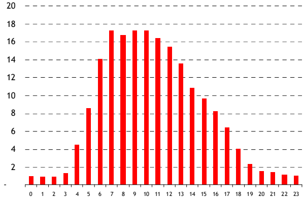
Profilo "artigiano" allacciato in BT (70MWh/anno) Profilo di consumo medio giornaliero (kWh)
