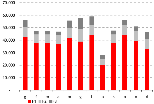
Profilo "impresa manifatturiera" allacciata in MT (600 MWh/anno) Profilo di consumo medio mensile (kWh)
